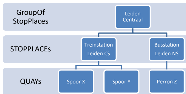
Figuur 3: Hiërarchie GroupOfStopPlaces, StopPlaces en Quays
