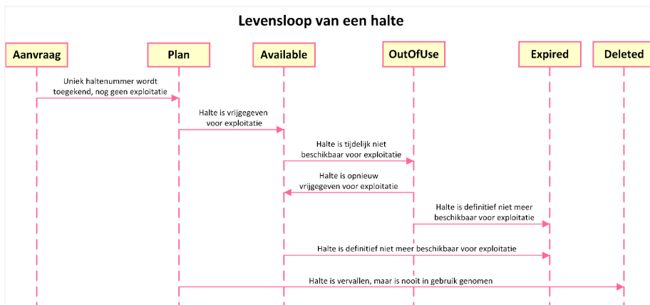
Figuur 4 Statusovergangen van een Quay
